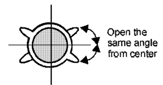
Vertical raster shift tabs
